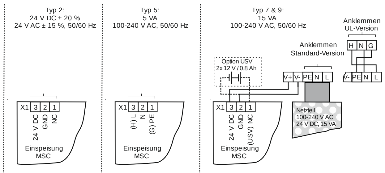
Abbildung 1: Anschluss Betriebsspannung
