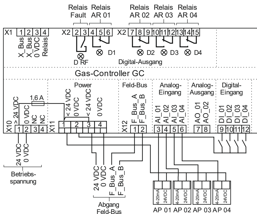
Abbildung 3: Anschlussschema
