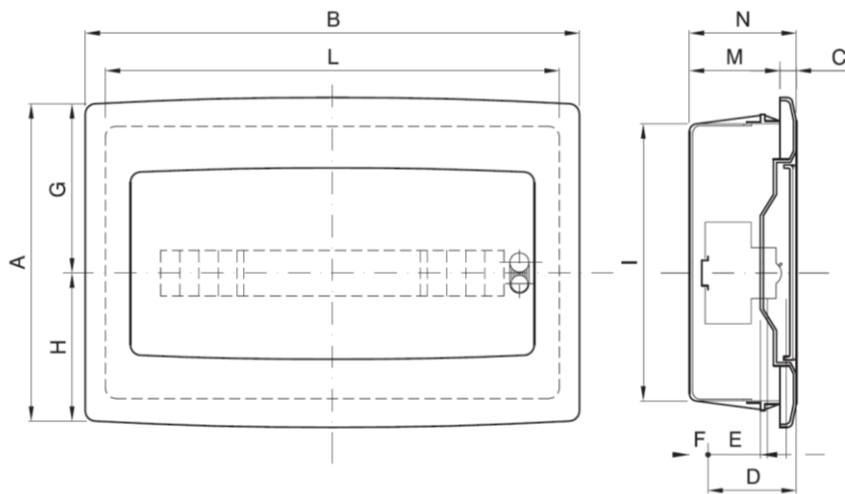
Abbildung 4: Abmessungen Türeinbau
